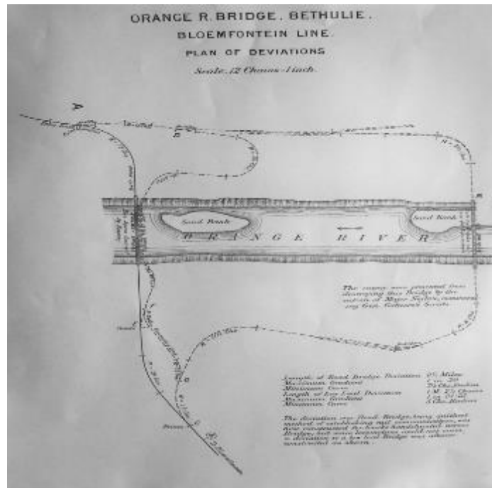
Skets van die spoorlyn wat oor die Bethulie-wabrug herlei is, 1900.
