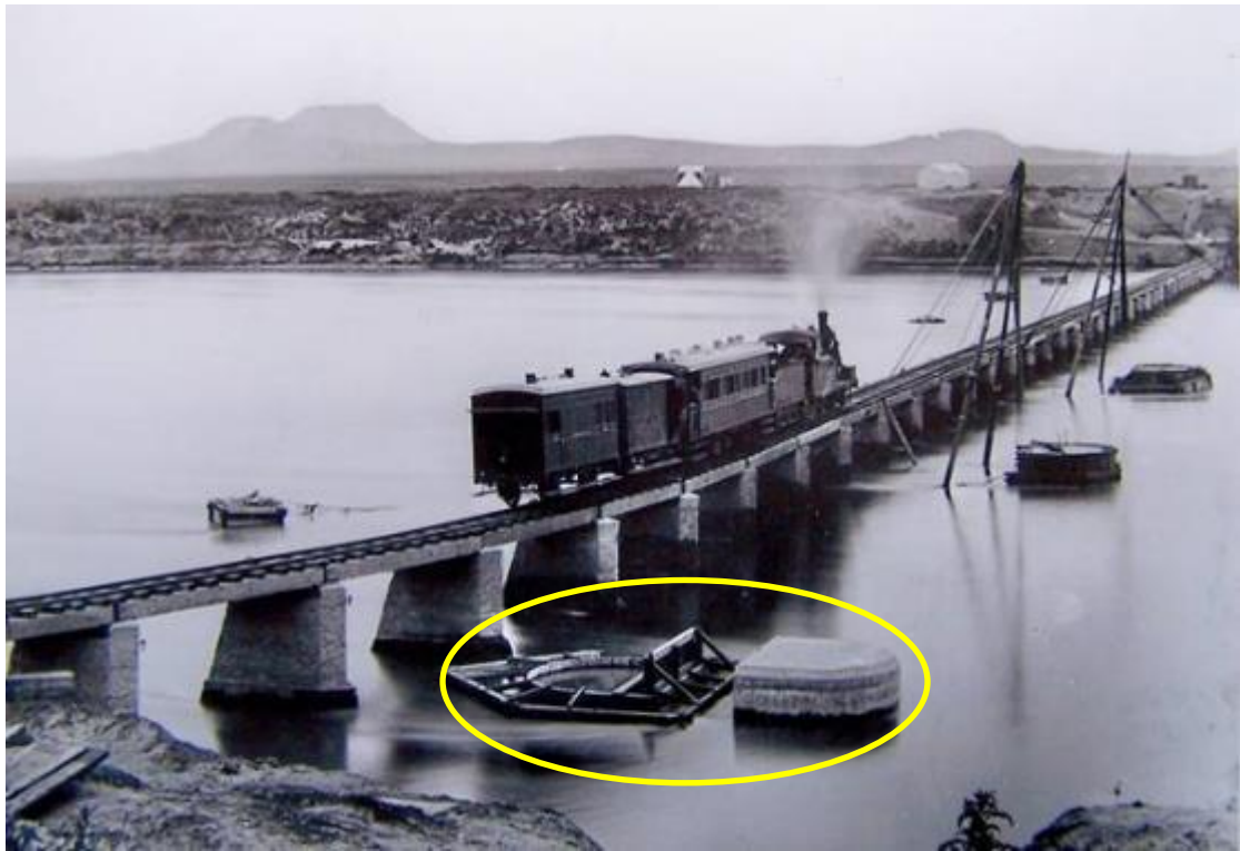
Die Bethulie-spoorbrug in aanbou, met die tydelike spoorbrug langs die voetstukke (1893). Bron: Oorlogsmuseum van die Boererepublieke, Bloemfontein.
