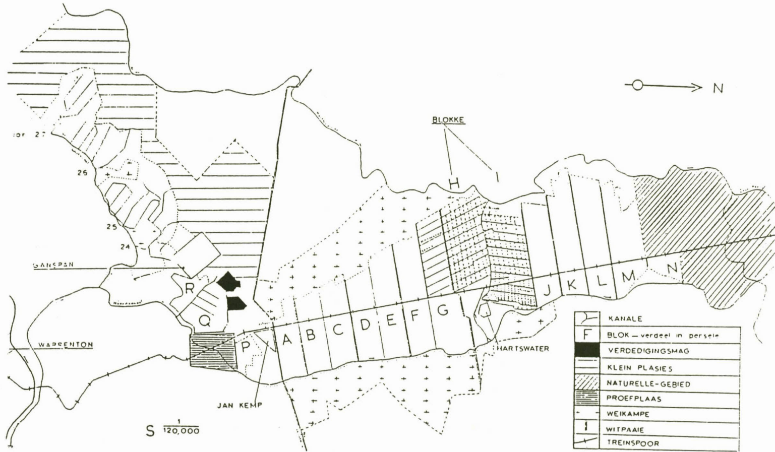
KAART 7: SKEMATIESE VOORSTELLING VAN VAALHARTSBESPROEING-SKEMA
